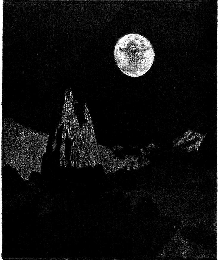
चित्र ३७—चन्द्रमा का एक दृश्य
